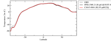
taszon
