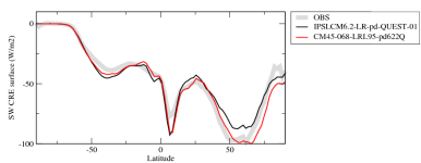
creltszon
