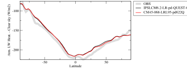
rlahcszone
