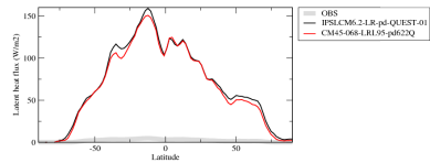
hfslszon
