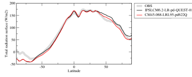
rtszon
