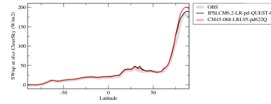
rsusczone
