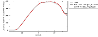
rsttcszone
