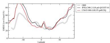
cllzon
