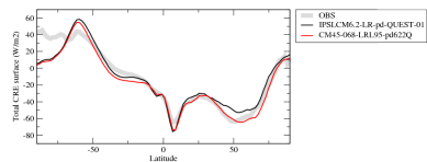
crettszon
