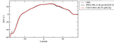
sstzon
