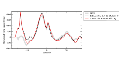
tauvzon
