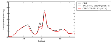
przon
