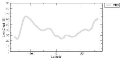
chlcalipsozon
