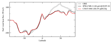
hfnszon
