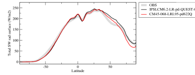
rstsczone
