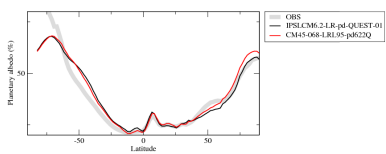
albtzon
