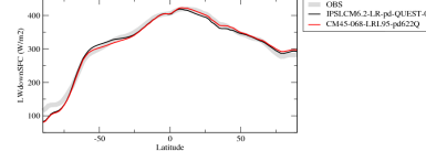
rldsczone
