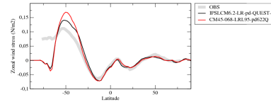
tauuzon
