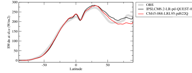
rsdsczone
