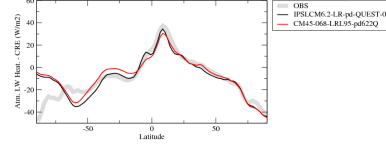
rlahcrezone
