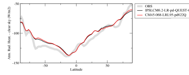
rahcszone
