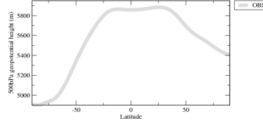
zg500zon
