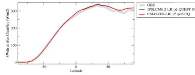
rsdscszone
