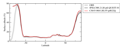
albszon
