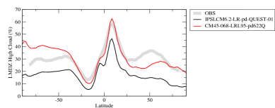
chlhzon
