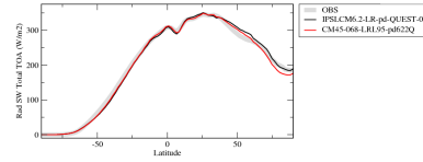
rsttzone
