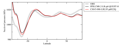
pslzon
