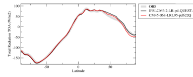
rttzn
