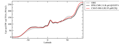
rsutzone
