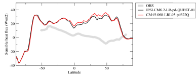
hfsszon
