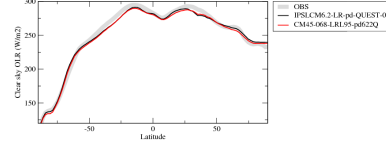
rlutcszone
