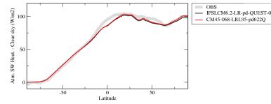
rsahcszone
