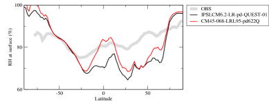
hurszon
