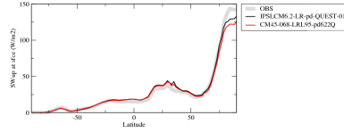
rsuszone
