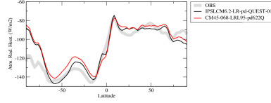
rahzon
