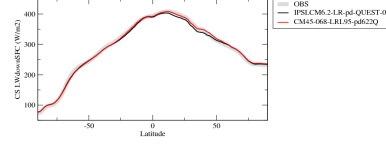
rldscszone
