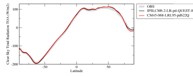
rttcszon
