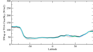
rsutszone
