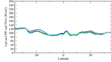
rsutzone
