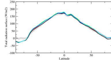
rtszone
