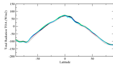
rttzone
