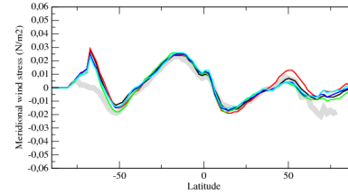
tauvzone
