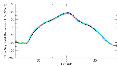
rttcszone
