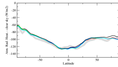
rahcszon
