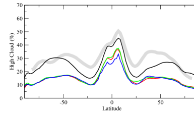
clhcalipsozon
