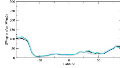
rsuszone
