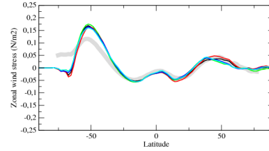
tauuzone
