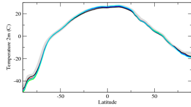
taszone
