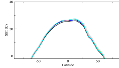
sstzone
