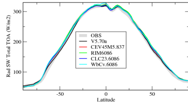
rsttzone
