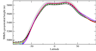
zg500zn
