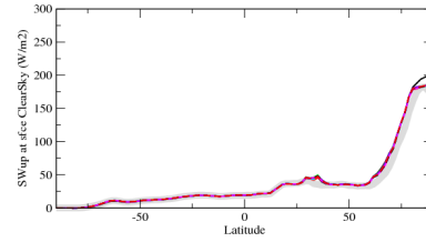
rsusczn
