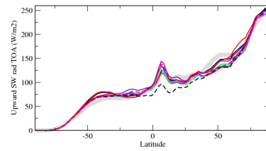
rsutzcn
