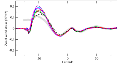
tauuzcn
