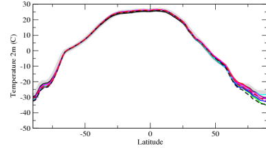
taszone
