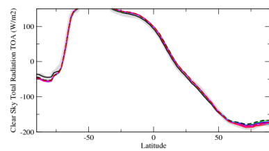
rttcszone
