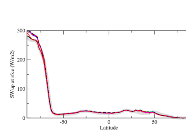
rsuszone
