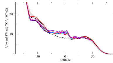
rsutzone
