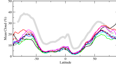
clmcalipsozon
