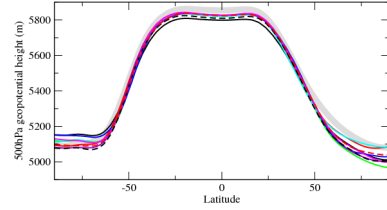
zg500zone
