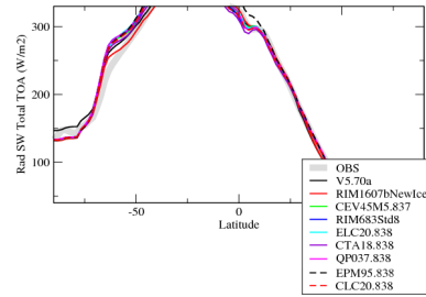
rsttzone
