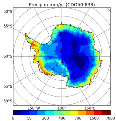
precipSH-CDO50-833
