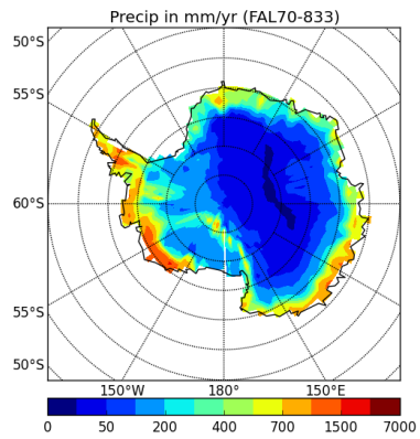
precipSH-FAL70-833
