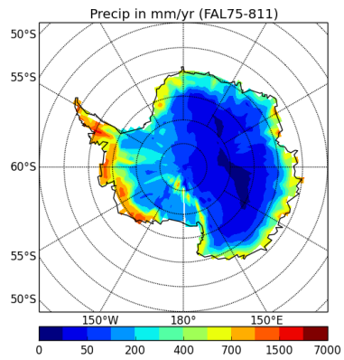
precipSH-FAL75-811
