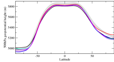
zg500zon
