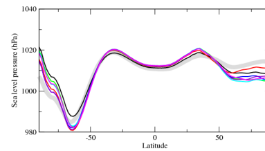
pslazon
