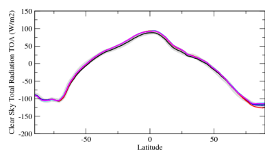
rttcszon
