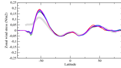
tauzon
