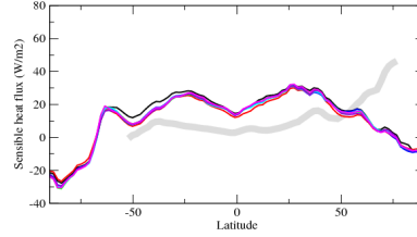
hfnlazon
