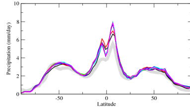
prazon
