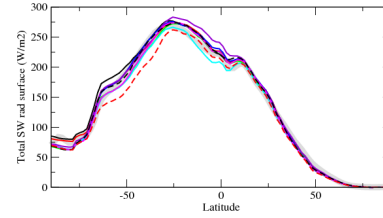
rstazon
