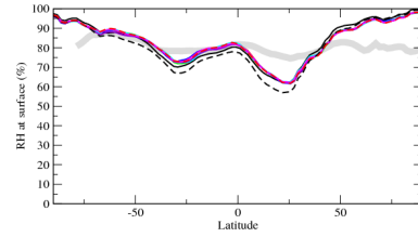
hurszone
