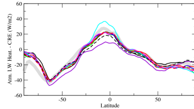
rlahcrezone
