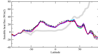
hfsszone
