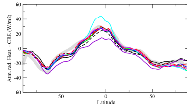
rahcrezone
