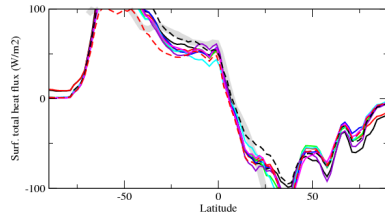
hfnszone
