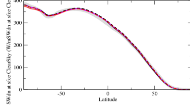
rsdscsazon
