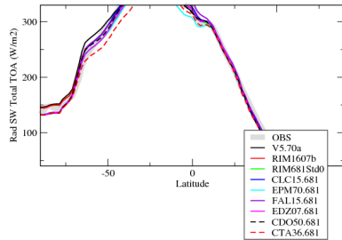
rsttazon
