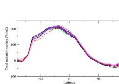
rtszon
