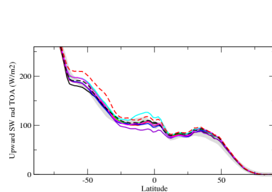
rsutzon
