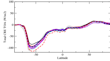
crettzn
