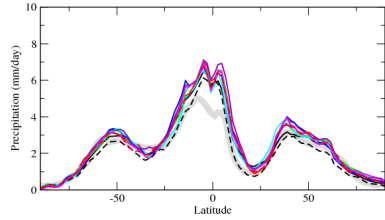
przone
