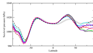
pslzone
