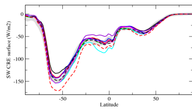
crosszon
