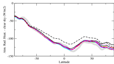
rahcszone
