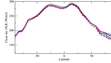
rlutszon
