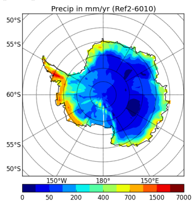
precipSH-Ref2-6010
