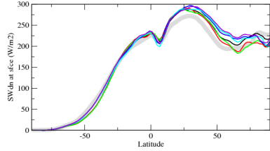
rsdszon
