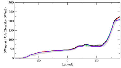
rsutczn
