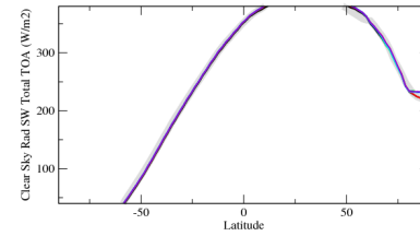
rsttcszon
