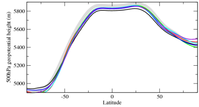
zg500zn
