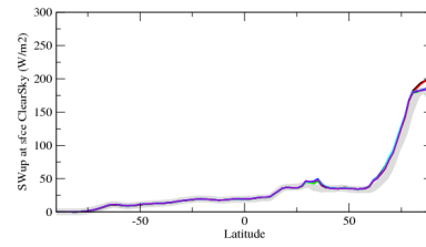
rsusczn
