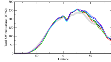
rstszon
