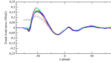
tauuzn
