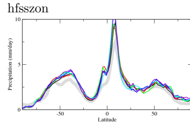
przon
