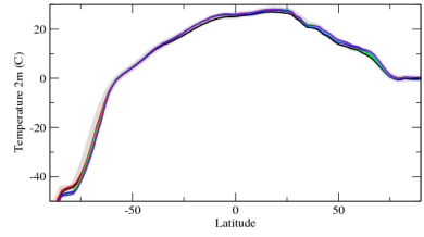
taszn
