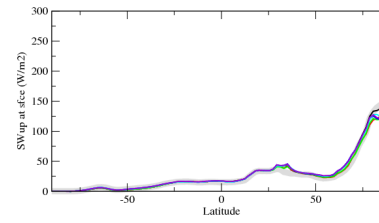
rsuszn
