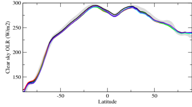
rlutcszon
