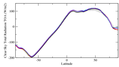
rttczn
