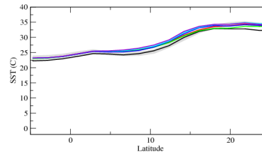
sstzn
