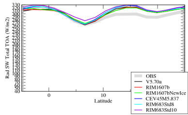
rsttzn
