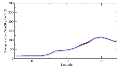
rsusczn
