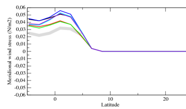
tauvzn
