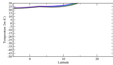
taszn
