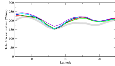
rstscszon
