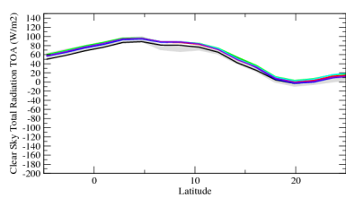
rttsczn
