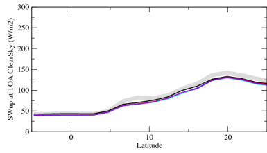
rsutsczn
