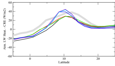
ralahcrezon
