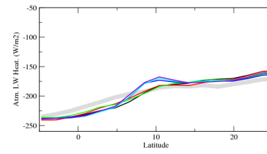
ralahzon
