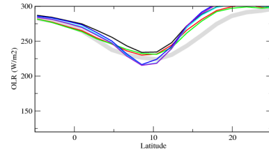
rlutscszon
