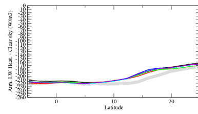
ralahcszon
