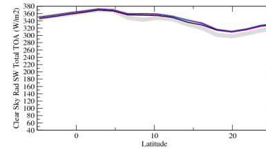
rsttscszon
