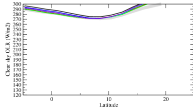
rlutscszon
