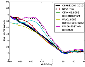
cretl_Tun6086
