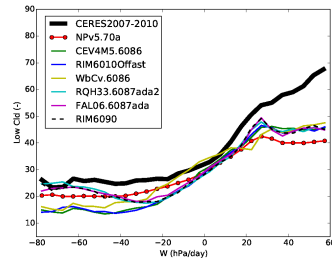
cllcalipso_Tun6086
