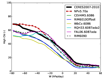
clhcalipso_Tun6086
