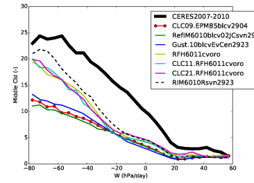
clmcalipso_Tun6011cvoro
