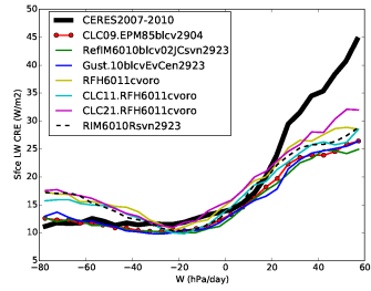
crels_Tun6011cvoro
