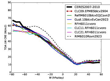
cretl_Tun6011cvoro
