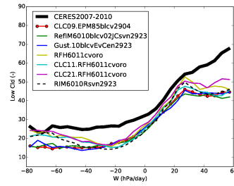
cllcalipso_Tun6011cvoro
