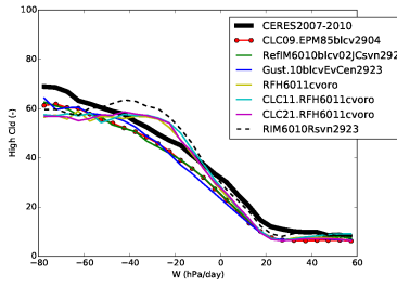
clhcalipso_Tun6011cvoro
