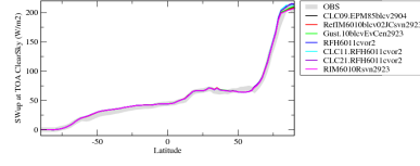
rsutcrezon
