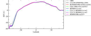
sstcrezon
