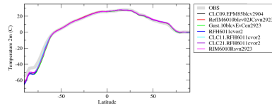
taszon
