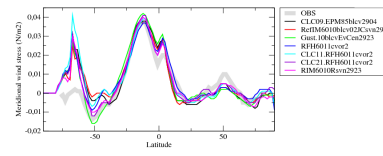
tauvzon
