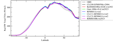
rsttcrezon
