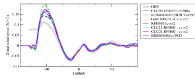
tauuzon
