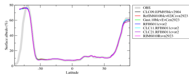
abszon
