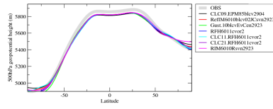
zg500zon
