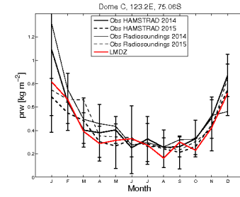
prw_DC_RadCv2Fiz.RIV104.1
