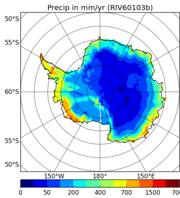
precipSH-RIV60103b
