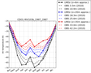
tempDC-CDO1-RIV103b_1987_1987
