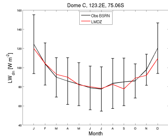
LWdnSFC_DC_CLC06.FAL0610_1987_1987
