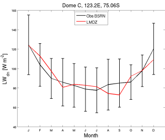
LWdnSFC_DC_CLC09.FAL0610_1987_1987
