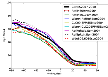
clhcalipso_Tun10wbrqh
