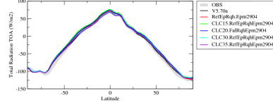
rttzn
