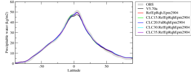
prwzon
