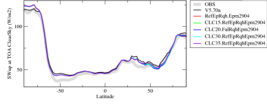
rsuteszon
