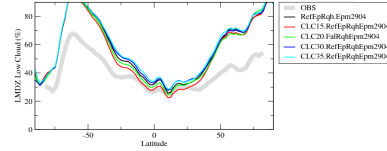
cllzon
