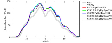
hflszon
