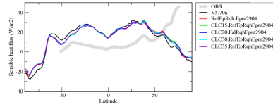
hfsszon
