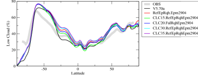
cllcalipsozon
