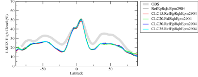
alhzon
