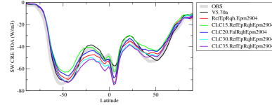
crestzn
