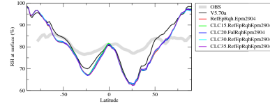
hurszon
