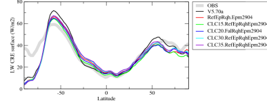
crelson
