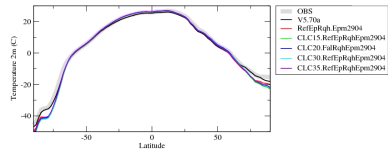
taszon
