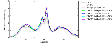
przon
