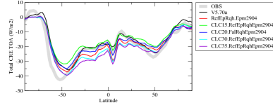
crettzn
