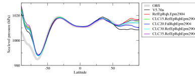
pslzon
