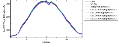
rsttzon
