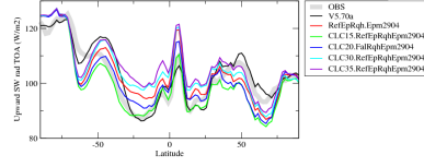
rsutzon
