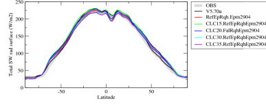
rstszon
