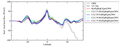
hfnszon
