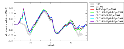
tauvzon
