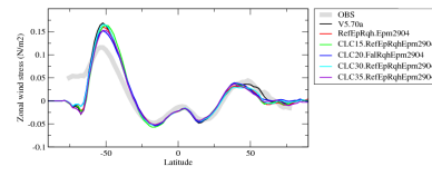
tauuzon
