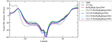
cretlzon
