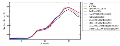
albszson
