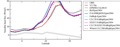
przson
