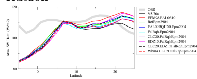
rsahszon
