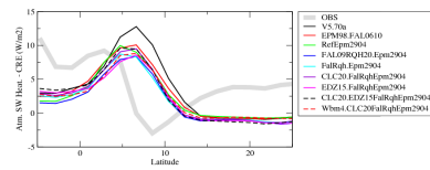
rlsruon
