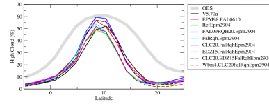
chlcalipsozon
