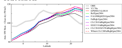
rsahcrezon
