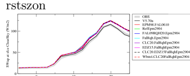
rstscszon
