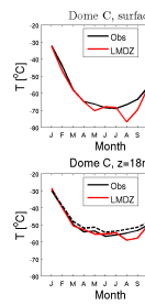
temp_DC_Re...
