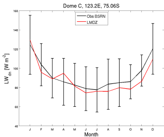
LWdnSFC_DC_RFH6010Isvn2923_1987_1987
