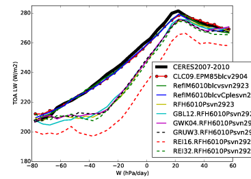
rlut_Tun10FHPrqhp
