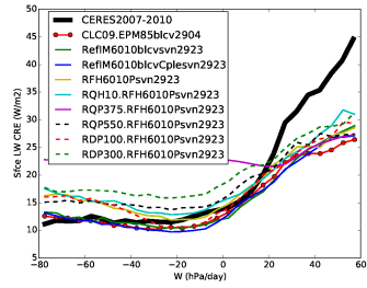
crels_Tun10FHPrqhp
