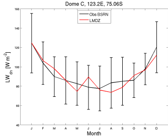
LWdnSFC_DC_RDP100.RFH6010Psvn2923_1987_1987
