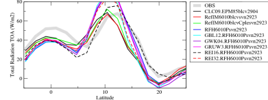
rttczon
