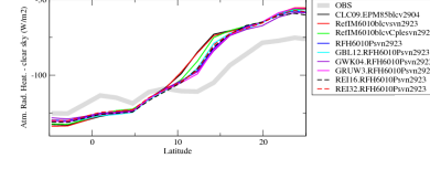
rahcszon
