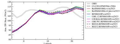
rsahczon
