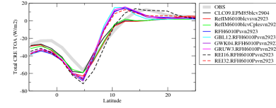
cretzon
