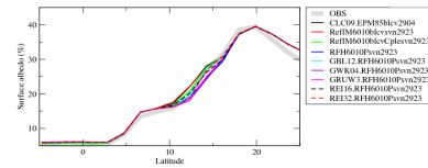
abszon
