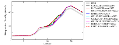
rsttczon
