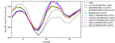
rsttcrezon
