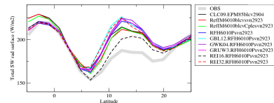
rsdczon
