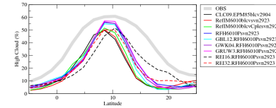
chlcalipsozon
