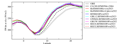
rsdcrezon
