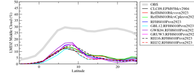
clmzon
