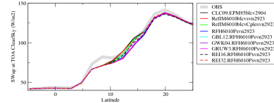
rsutcrezon
