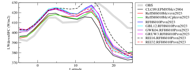
rldczon
