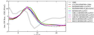
rsahzon
