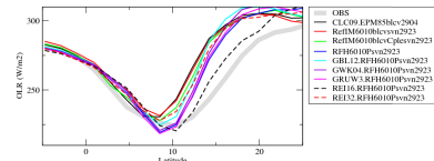
rlutczon
