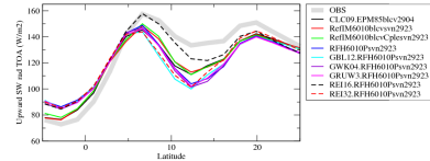
rsutczon
