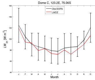
LWdnSFC_DC_FAL07.RFH6010Psvn2923.1987_1987
