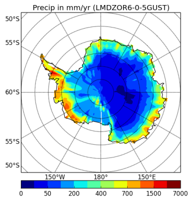
precipSH-LMDZOR6-0-5GUST
