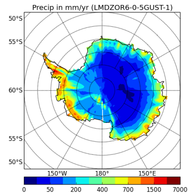
precipSH-LMDZOR6-0-5GUST-1
