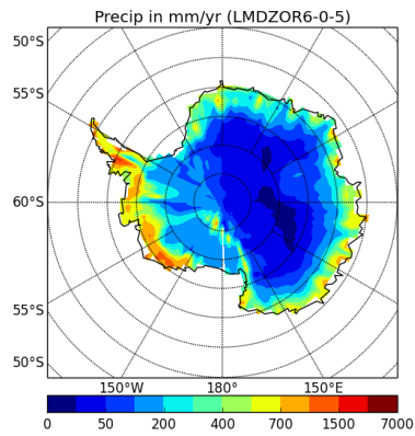
precipSH-LMDZOR6-0-5
