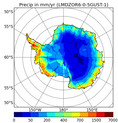
precipSH-LMDZOR6-0-5GUST-1
