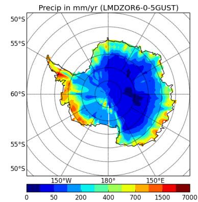
precipSH-LMDZOR6-0-5GUST
