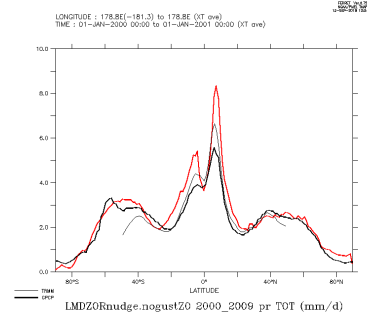
LMDZORnudge.nogustZ0_2000_2009_tot
