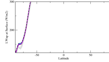
rluszone
