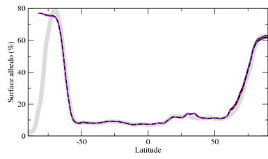
albszon
