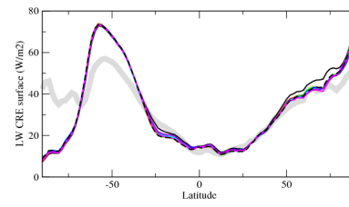
crelszon
