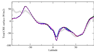
cretzon
