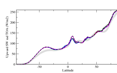
rsutzone
