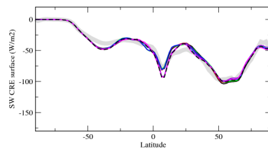
cresszon
