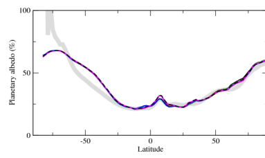
albtzon
