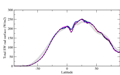
rstszone
