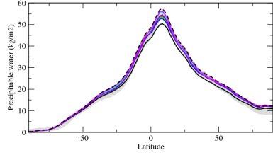
prwzon
