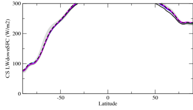
rldscszon
