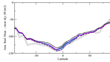
rahcszon
