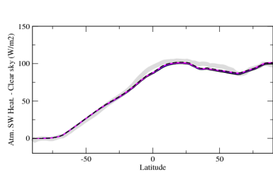
rsahcszon
