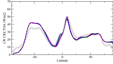
creltzon
