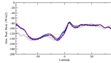
rahzon
