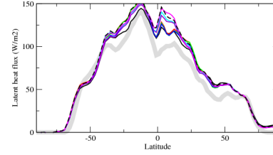
hfhszon
