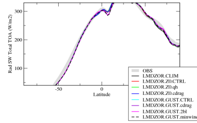
rstszone
