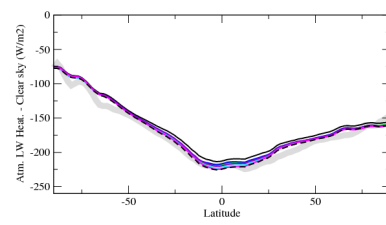
rlahcszon
