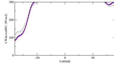
rldszone
