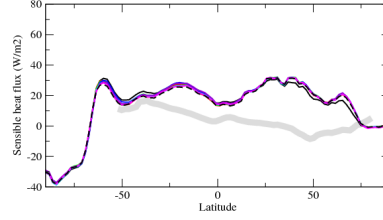
hfsszon
