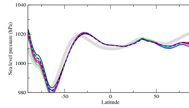
pslzon
