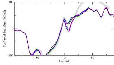
hfmszon
