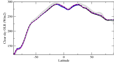
rlutcszon
