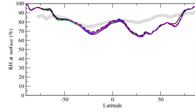
hurszon
