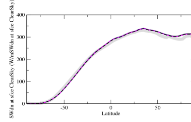
rsdscszon
