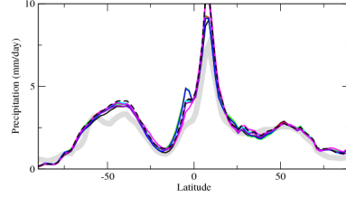
przon
