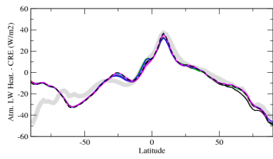
rlahcrezon
