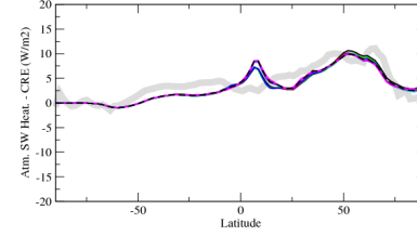
rsahcrezon
