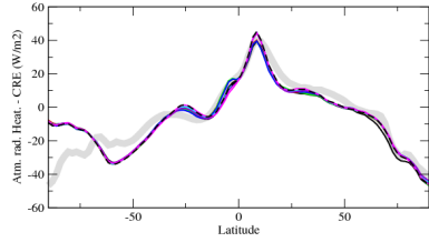
rahcrezon
