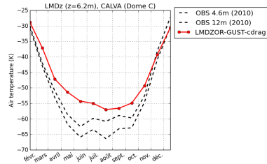
tempDC-LMDZOR-GUST-cdrag
