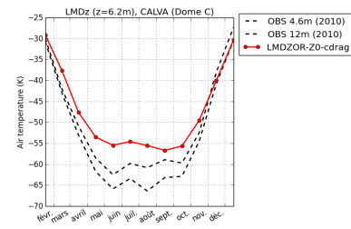
tempDC-LMDZOR-Z0-cdrag
