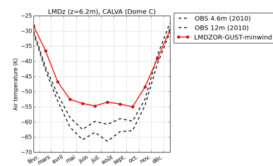
tempDC-LMDZOR-GUST-minwind
