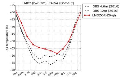
tempDC-LMDZOR-Z0-qh
