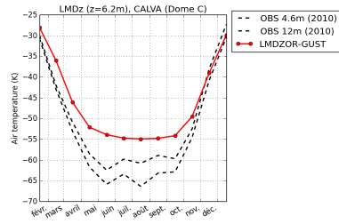
tempDC-LMDZOR-GUST
