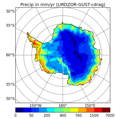
precipSH-LMDZOR-GUST-cdrag
