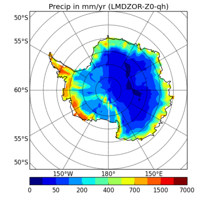
precipSH-LMDZOR-Z0-qh
