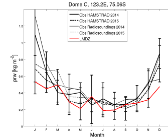
prw_DC_LMDZ.REF_1980_1980
