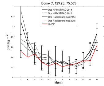
prw_DC_LMDZ.16OMP_1980_1980
