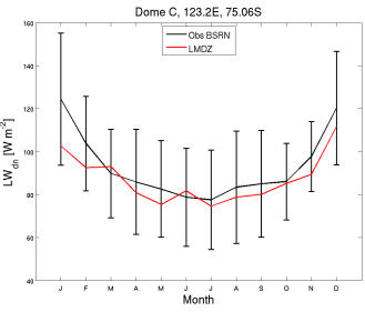
LWdnSFC_DC_LMDZ.16OMP_1980_1980
