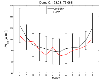
LWdnSFC_DC_LMDZ.REF_1980_1980
