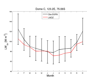
LWdnSFC_DC_LMDZ.12OMP_1980_1980
