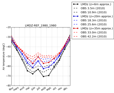
tempDC-LMDZ-REF_1980_1980
