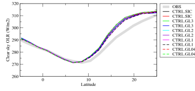
rlutazon
