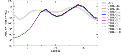
rsahzon
