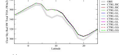
rsttcsazon
