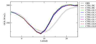
rlutazon
