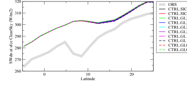
rsdscsazon
