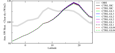
rsahcsazon
