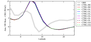
rsahcrezon
