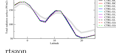
rtsazon
