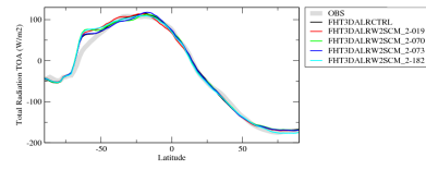
rttzn
