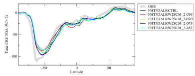
cretzon
