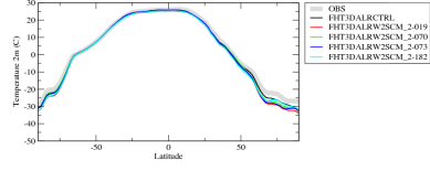
taszn
