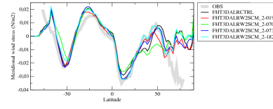
tauvzn
