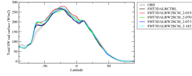
rstsczon
