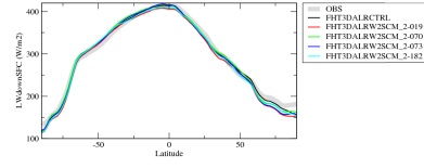
rldsczon
