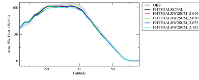
rsahazon
