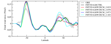
tauuzn
