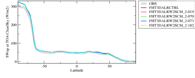
rsutscszon
