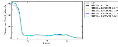
rsuscsczon
