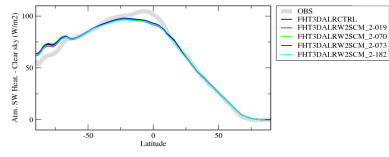
rsahscszon
