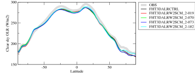
rlutscszon
