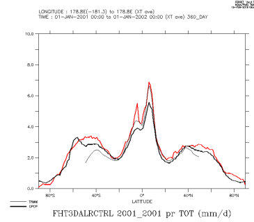
FHT3DALRCTRL_2001_2001_tot
