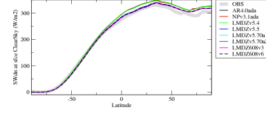
rsdscszone
