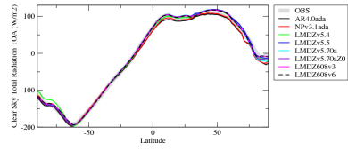
rtteszon
