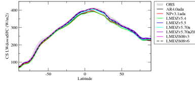
rldscszone
