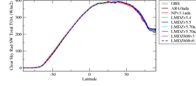
rsttcszone
