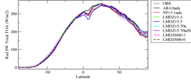
rsttzone
