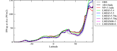
rsuszone
