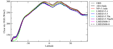
rlutcszone
