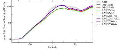
rsahcszone
