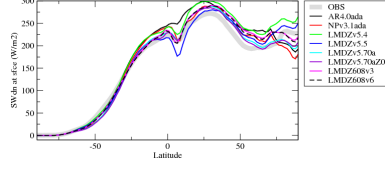
rsdszone
