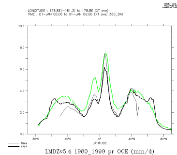
LMDZv5.4_1980_1999_oce
