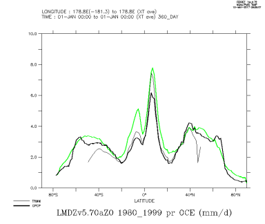
LMDZv5.70aZ0_1980_1999_oce
