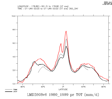
LMDZ608v6_1980_1999_tot
