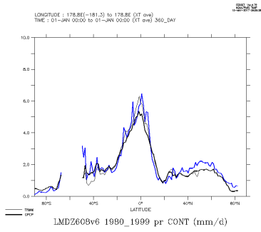
LMDZ608v6_1980_1999_con
