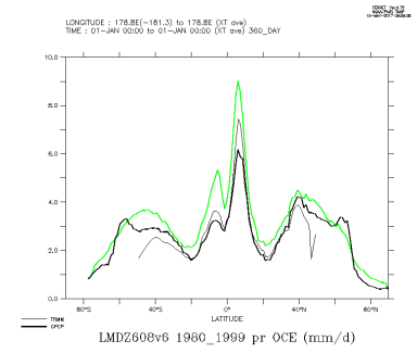
LMDZ608v6_1980_1999_oce
