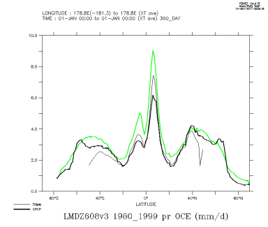
LMDZ608v3_1980_1999_oce
