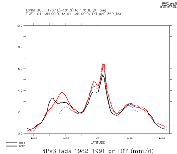
NPv3.1ada_1982_1991_tot
