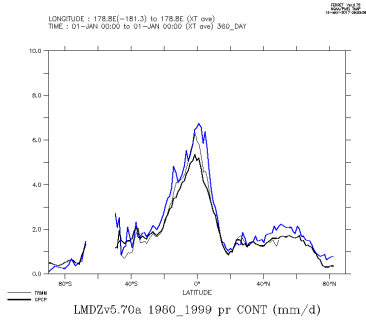
LMDZv5.70a_1980_1999_con
