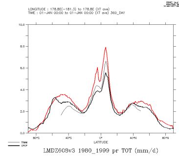
LMDZ608v3_1980_1999_tot
