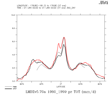
LMDZv5.70a_1980_1999_tot
