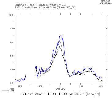
LMDZv5.70aZ0_1980_1999_con
