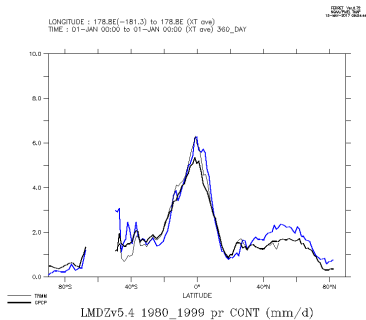
LMDZv5.4_1980_1999_con
