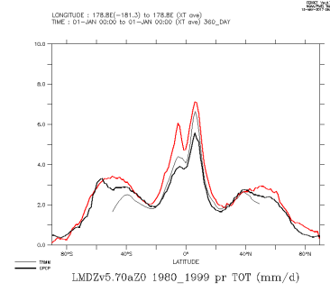
LMDZv5.70aZ0_1980_1999_tot
