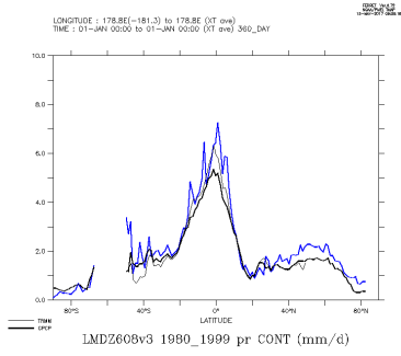
LMDZ608v3_1980_1999_con
