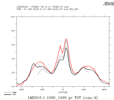
LMDZv5.4_1980_1999_tot
