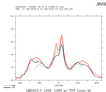
LMDZv5.5_1980_1999_tot
