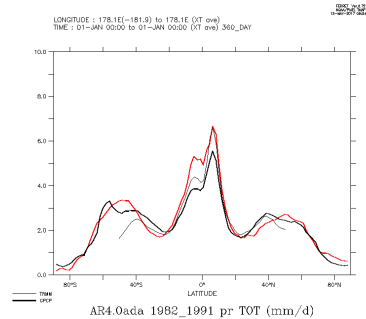
AR4.0ada_1982_1991_tot
