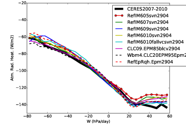
rah_RETRO5TO10
