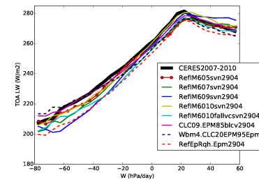
rlut_RETRO5TO10
