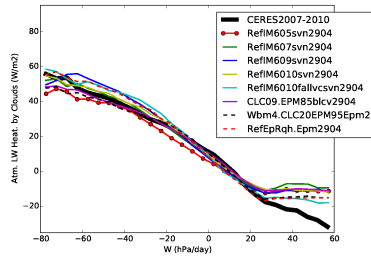
rlahcre_RETRO5TO10
