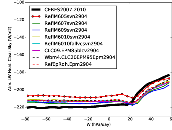
rlahcs_RETRO5TO10
