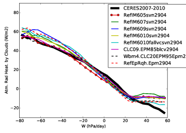
rahcre_RETRO5TO10
