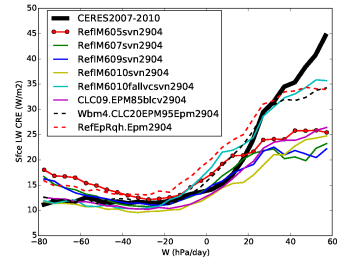
crels_RETRO5TO10
