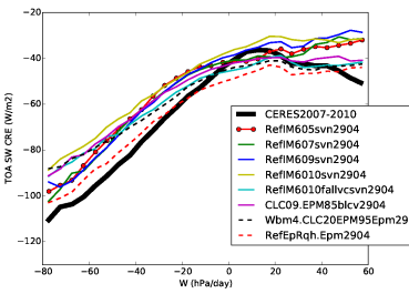
crest_RETRO5TO10
