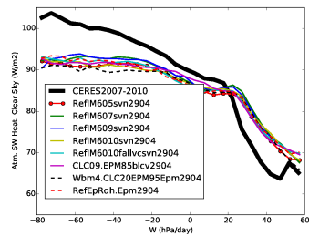
rsahcs_RETRO5TO10
