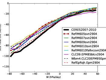
crets_RETRO5TO10
