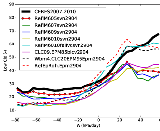
cllcalipso_RETRO5TO10
