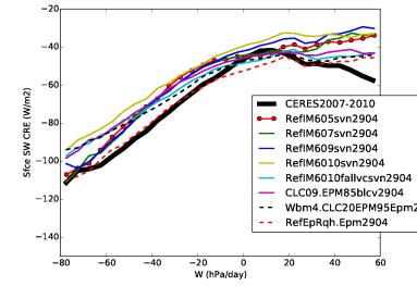
cross_RETRO5TO10
