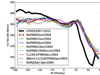
rsttcs_RETRO5TO10
