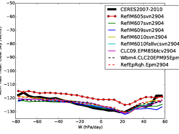
rahcs_RETRO5TO10
