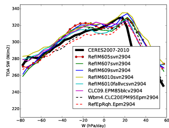
rstt_RETRO5TO10
