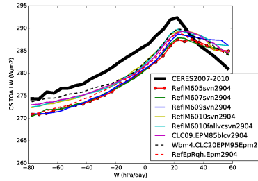
rlutcs_RETRO5TO10
