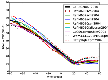
cretl_RETRO5TO10
