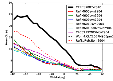
clmcalipso_RETRO5TO10
