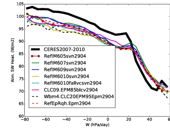
rsah_RETRO5TO10
