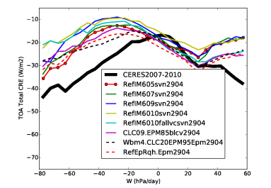
crett_RETRO5TO10
