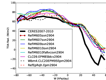
rtt_RETRO5TO10
