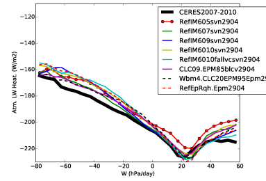
rlah_RETRO5TO10
