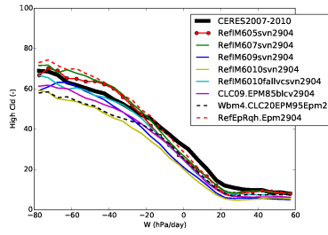
clhcalipso_RETRO5TO10
