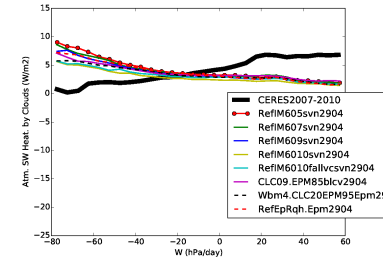
rsahcre_RETRO5TO10
