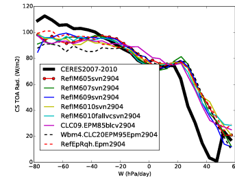
rttcs_RETRO5TO10
