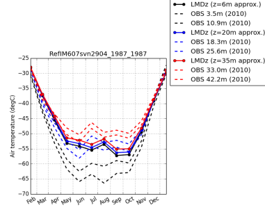
tempDC-RefIM607svn2904_1987_1987
