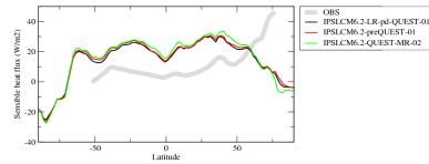
hfnsszon
