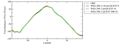
rttzon
