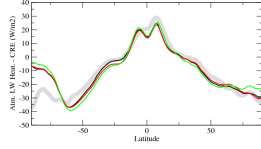
rlahcrezon
