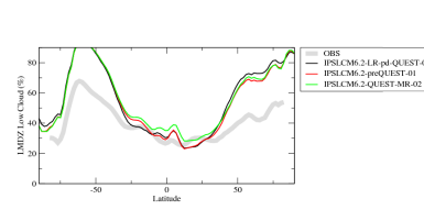
cllzozon
