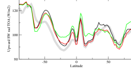
rsutzon
