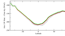
rldscszon
