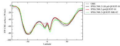
cresslzon
