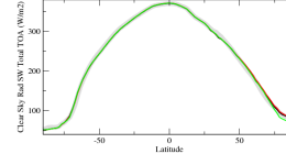
rsttcszon
