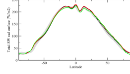
rstcszon
