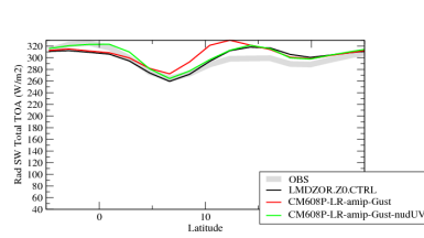
rsttzn
