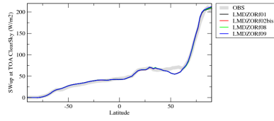
rsuteszon
