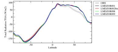
rtdscszon
