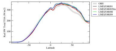
rsttazon
