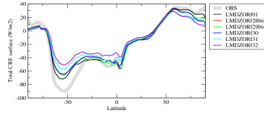
cretlzon
