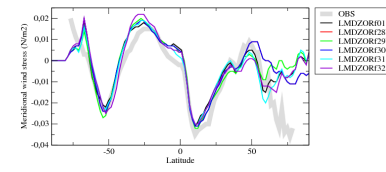
tauvzon
