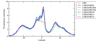
przon
