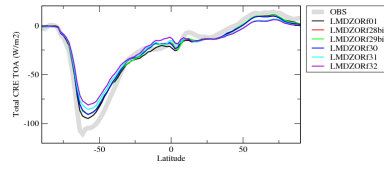
crettzon
