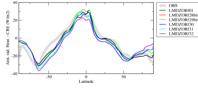
rahcrezon
