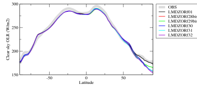
rlutcszon
