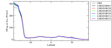
rsuszon
