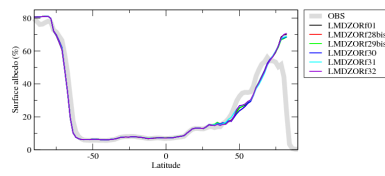
albszon
