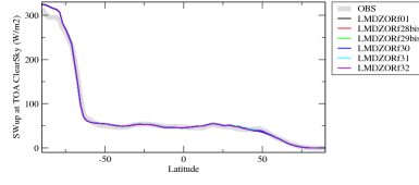
rsutcszon
