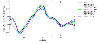
ralhcrezon
