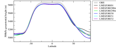
zg500zon
