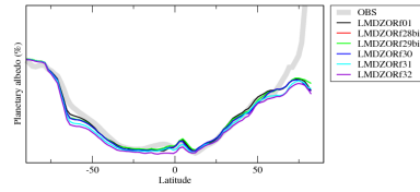
albtzon
