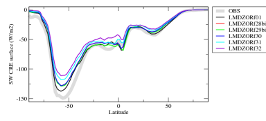
cretsszon
