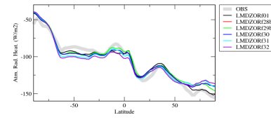
rahzon
