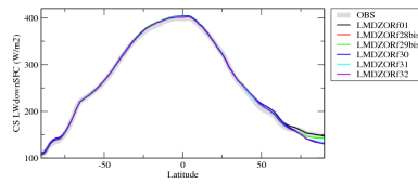
rldscszon
