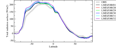
rtszon
