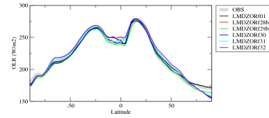
rlutazon
