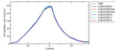
prwzon
