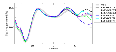
pslzon
