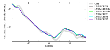
rahcszon
