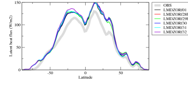
hflszon
