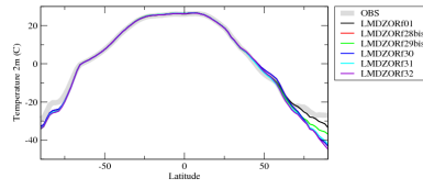
taszon
