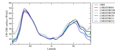
crelszon
