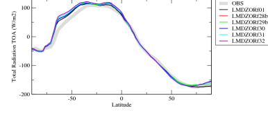
rttazon
