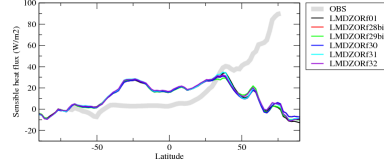
hfsszon
