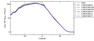
rsahazon
