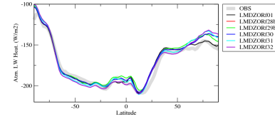
ralhzon
