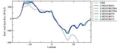
hfnszon
