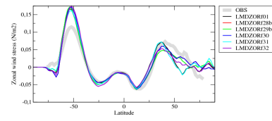
tauuzon
