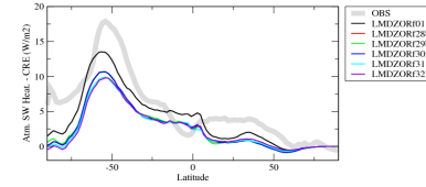
rsahrszon
