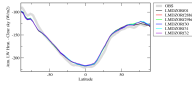
ralhcszon
