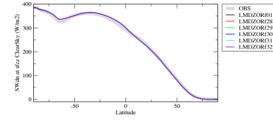
rsdsrszon
