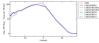
rsahcszon
