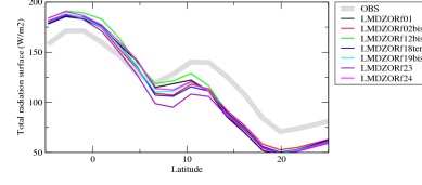
rsuscsczon
