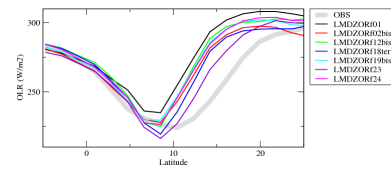
rlutsczon
