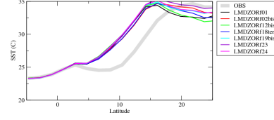
rttsczon
