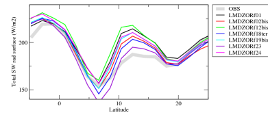
rsdsczon
