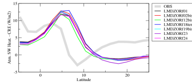
rlutsczon
