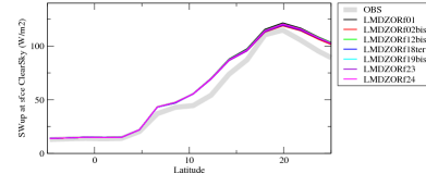
rsttsczon
