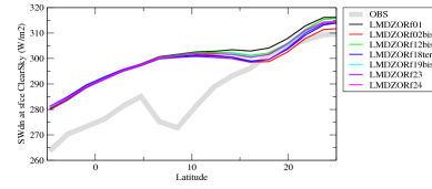
rsahsczon
