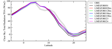
rttscszon
