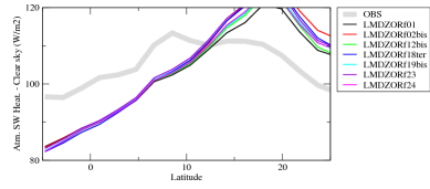
rsahscszon
