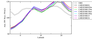
rsahsczon
