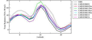
rttsczon
