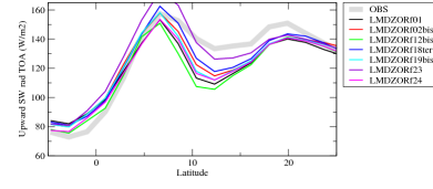
rsuscsczon
