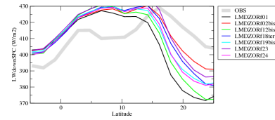
rldsczon
