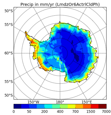
precipSH-LmdzOr6ActrlCldPh
