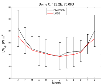
LWdnSFC_DC_LmdzOr6Actrl.1990_1999
