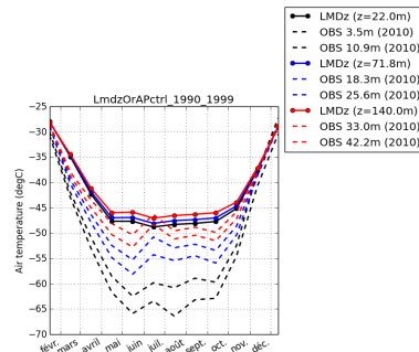
tempDC-LmdzOrAPctrl.1990_1999
