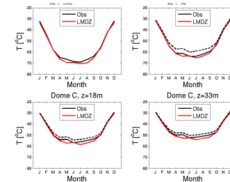
temp_DC_LmdzOr6Actrl.1990_1999
