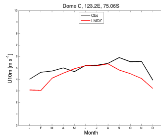
wind10m_DC_LmdzOrChoiAP.1990_1999
