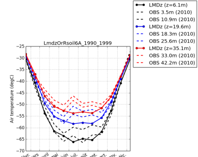
tempDC-LmdzOrRsoil6A_1990_1999
