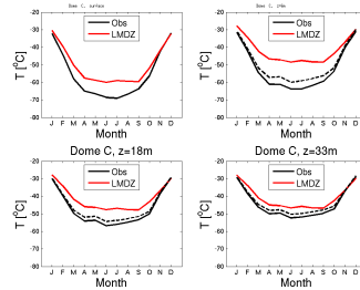
temp_DC_LmdzOrChoiAP.1990_1999
