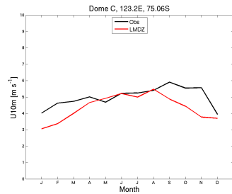
wind10m_DC_LmdzOrAPctrl.1990_1999
