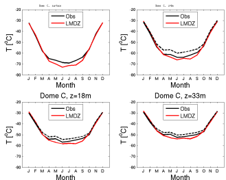
temp_DC_LmdzOrRsoil6A_1990_1999
