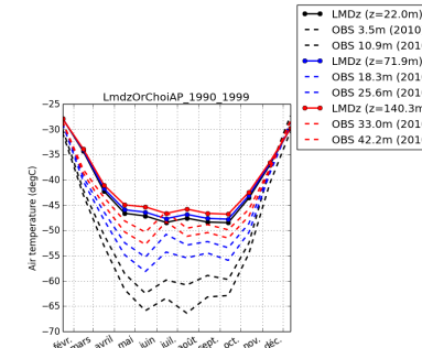
tempDC-LmdzOrChoiAP.1990_1999
