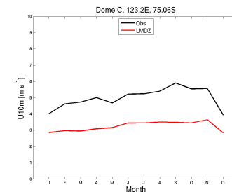
wind10m_DC_LmdzOr6Actrl.1990_1999
