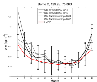
prw_DC_LmdzOr6Actrl.1990_1999
