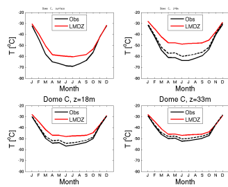
temp_DC_LmdzOrAPctrl.1990_1999
