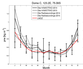
prw_DC_LmdzOrChoiAP.1990_1999
