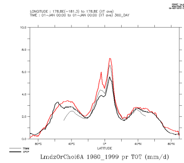
LmdzOrChoi6A_1980_1999_tot
