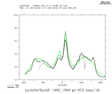
LmdzOrChoiAP_1980_1999_oce
