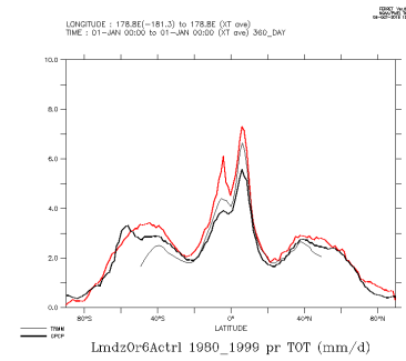
LmdzOr6Actrl_1980_1999_tot
