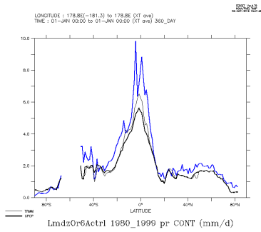
LmdzOr6Actrl_1980_1999_con
