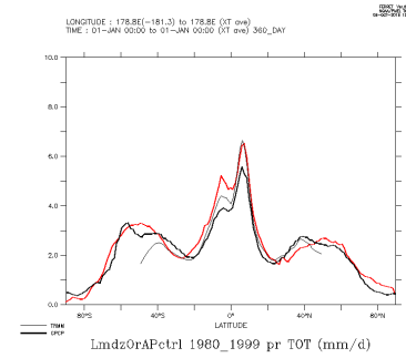
LmdzOrAPctrl_1980_1999_tot
