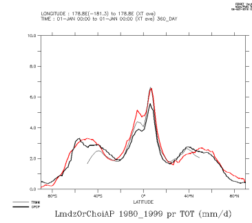
LmdzOrChoiAP_1980_1999_tot
