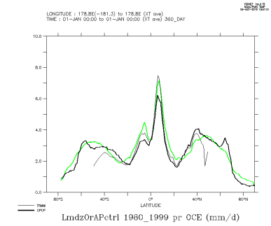
LmdzOrAPctrl_1980_1999_oce
