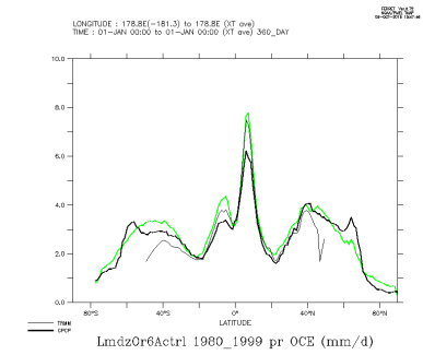
LmdzOr6Actrl_1980_1999_oce
