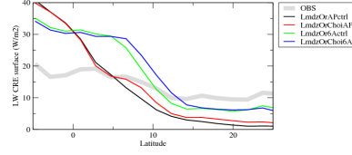
crelsson
