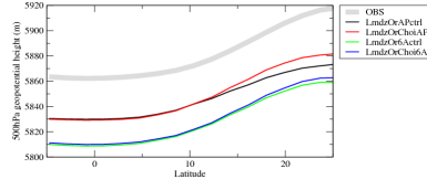
zg500zon
