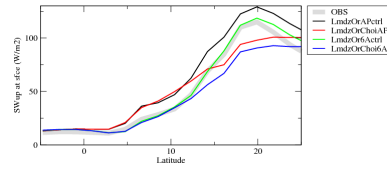
rstczon
