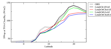
rsuteszon
