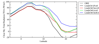
rttcson
