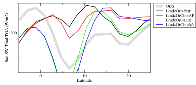
rsdsczon
