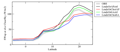
rstcszo
