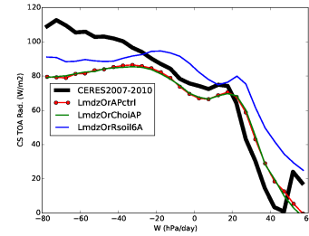
rttcs_LmdzOr11et2cAP
