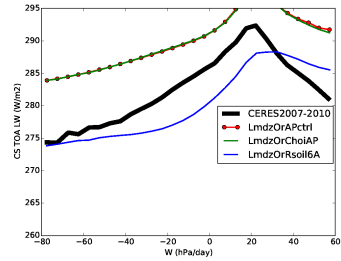
rlutcs_LmdzOr11et2cAP
