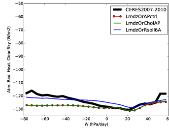
rahcs_LmdzOr11et2cAP
