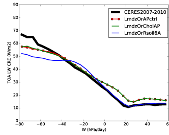
cretl_LmdzOr11et2cAP
