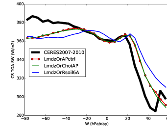
rsttcs_LmdzOr11et2cAP
