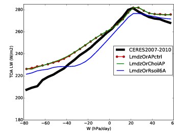
rlut_LmdzOr11et2cAP
