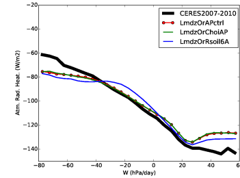
rah_LmdzOr11et2cAP
