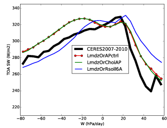
rstt_LmdzOr11et2cAP
