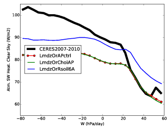
rsahcs_LmdzOr11et2cAP
