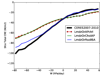
cretts_LmdzOr11et2cAP
