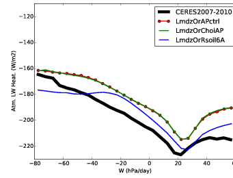
rlah_LmdzOr11et2cAP
