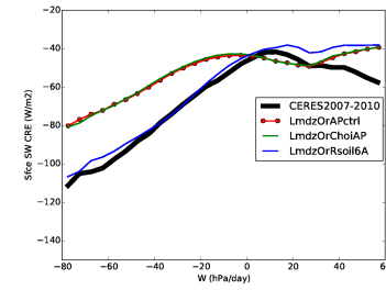
cress_LmdzOr11et2cAP
