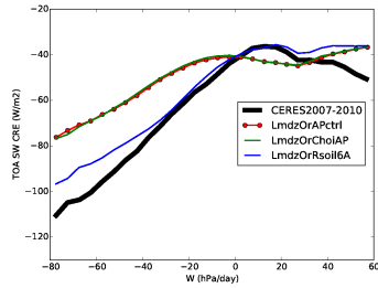
crest_LmdzOr11et2cAP
