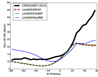
crels_LmdzOr11et2cAP
