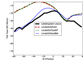
crettt_LmdzOr11et2cAP
