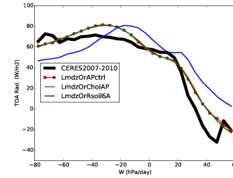
rtt_LmdzOr11et2cAP
