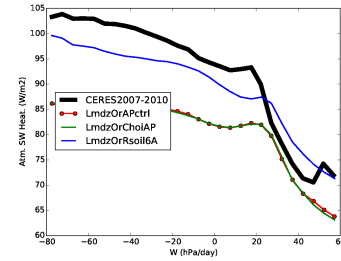
rsah_LmdzOr11et2cAP
